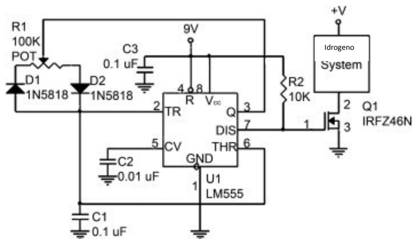
Figura. 1. Schema della centralina elettronica idrossi (HECU).
